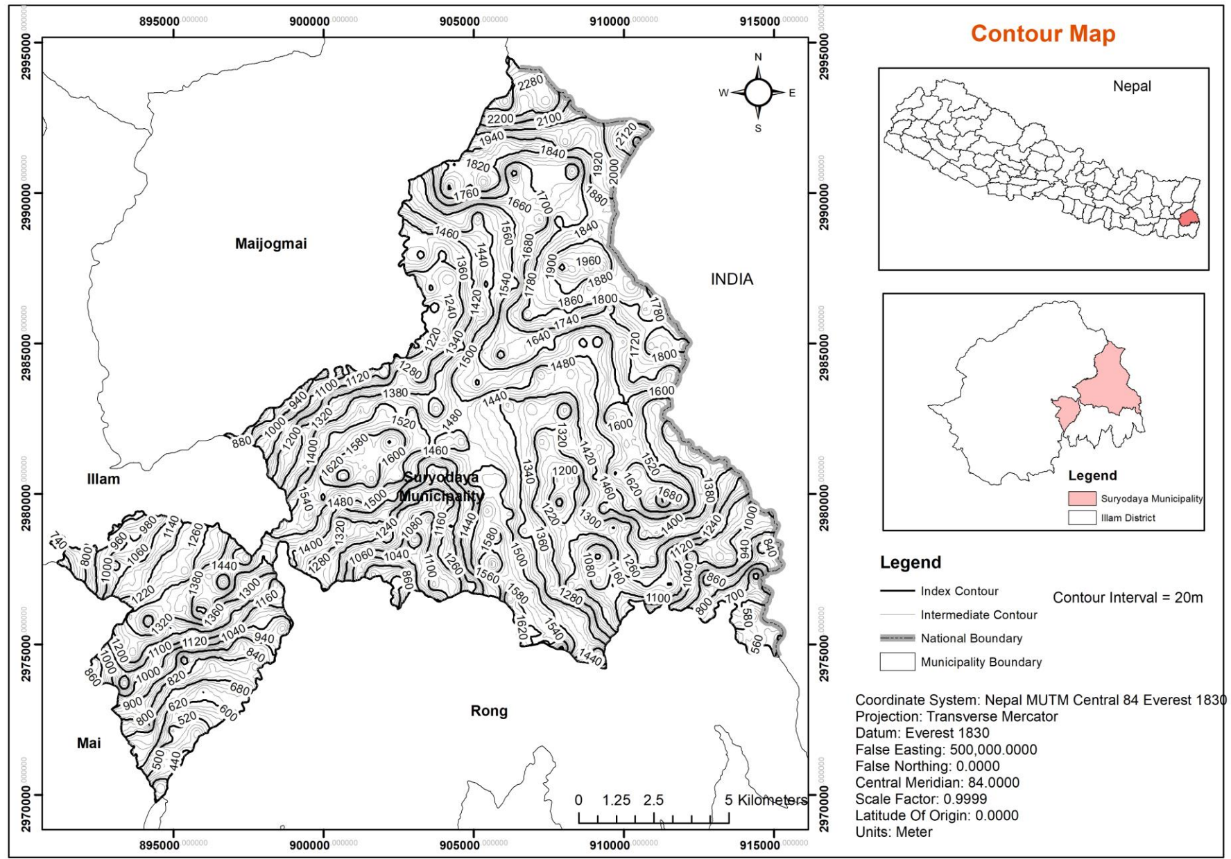
चित्र १६: सूर्योदय नगरपालिकाको कन्टोर नक्शा (Contour Map)
